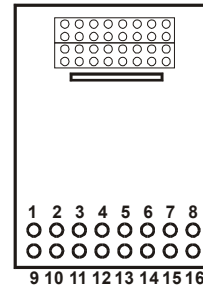
CH-Controller Ansicht gegen Stecker Connector View
