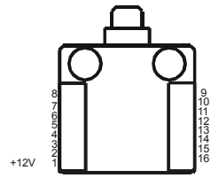
Ansicht auf Klemmen Screw terminal view
